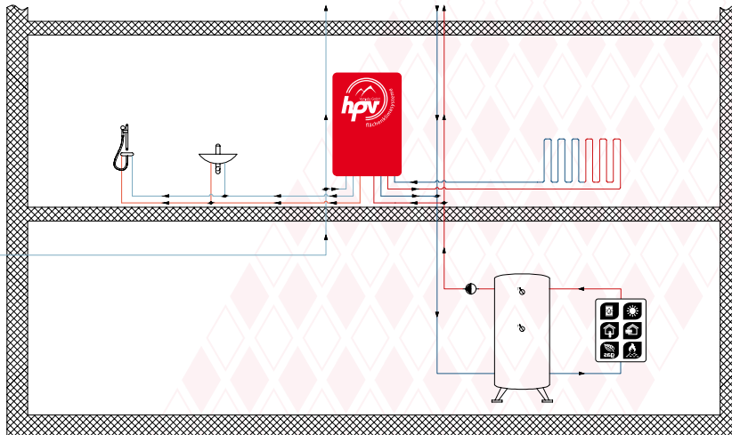
Frischwassersatz für Wohnungsübergabestation. Bausatz 2
